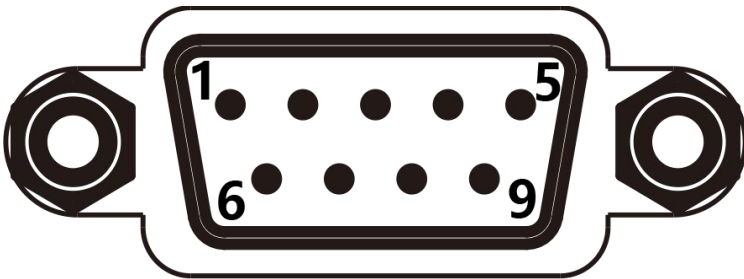
RS-232
